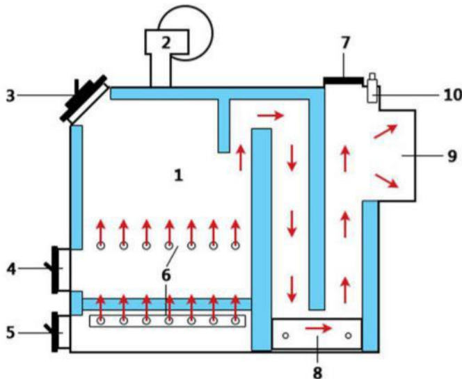
рис. 1 Конструкция котла
